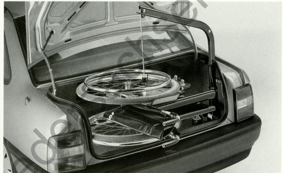
Elektrischer Rollstuhllifter für das Unterbringen des Rollstuhls im Kofferraum.
