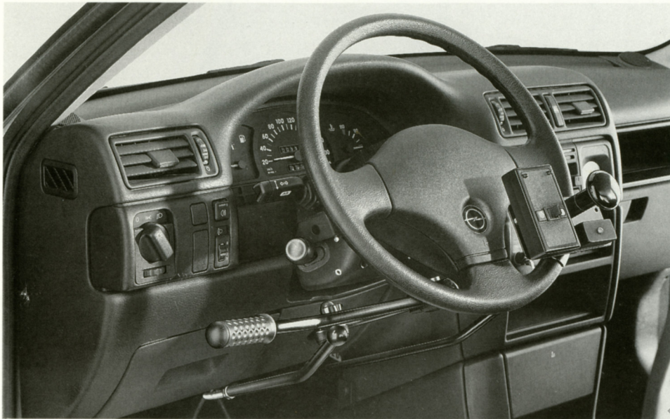
Handbedienung von Bremse und Gas. Lenkhilfe mit Zentral-Commander.
