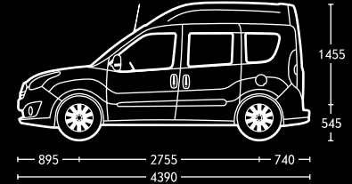
Combo mit Radstand L1 und Dachhöhe H2. 1
