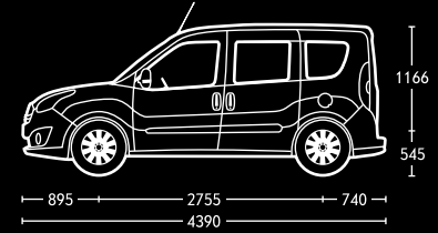
Combo mit Radstand L1 und Dachhöhe H1.
