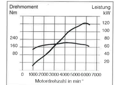
Souveräne Durchzugskraft: Der Vierventiler erreicht bei 4200 min -1 sein maximales Drehmoment von 227 Nm. Im Bereich zwischen 1600 und 6400 min -1 stehen beachtliche 180 Nm zur Verfügung.
