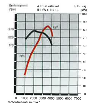
Der 3.1-Turbodiesel entwickelt sein maximales Drehmoment von 260 Nm bei 2.000 min -1 .
